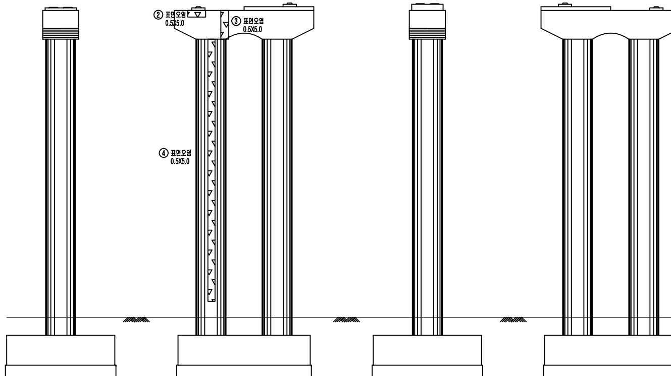
좌측면
